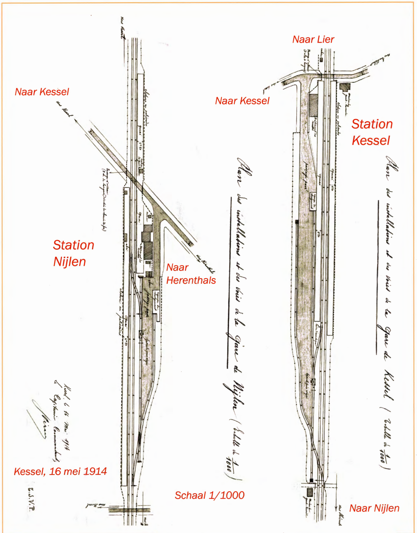
Gedetailleerde schetsen van de stations van Kessel en Nijlen, mei 1914. Alle strategisch belangrijk geachte infrastructuur werd in een lijvig schetsboek uitgetekend. Ten behoeve van onze lezers hebben wij de schetsen van de stations 90 graden gedraaid, waardoor een betere leesbaarheid bekomen werd. Op de schetsen bracht de redactie enkele aantekeningen in het rood aan.
