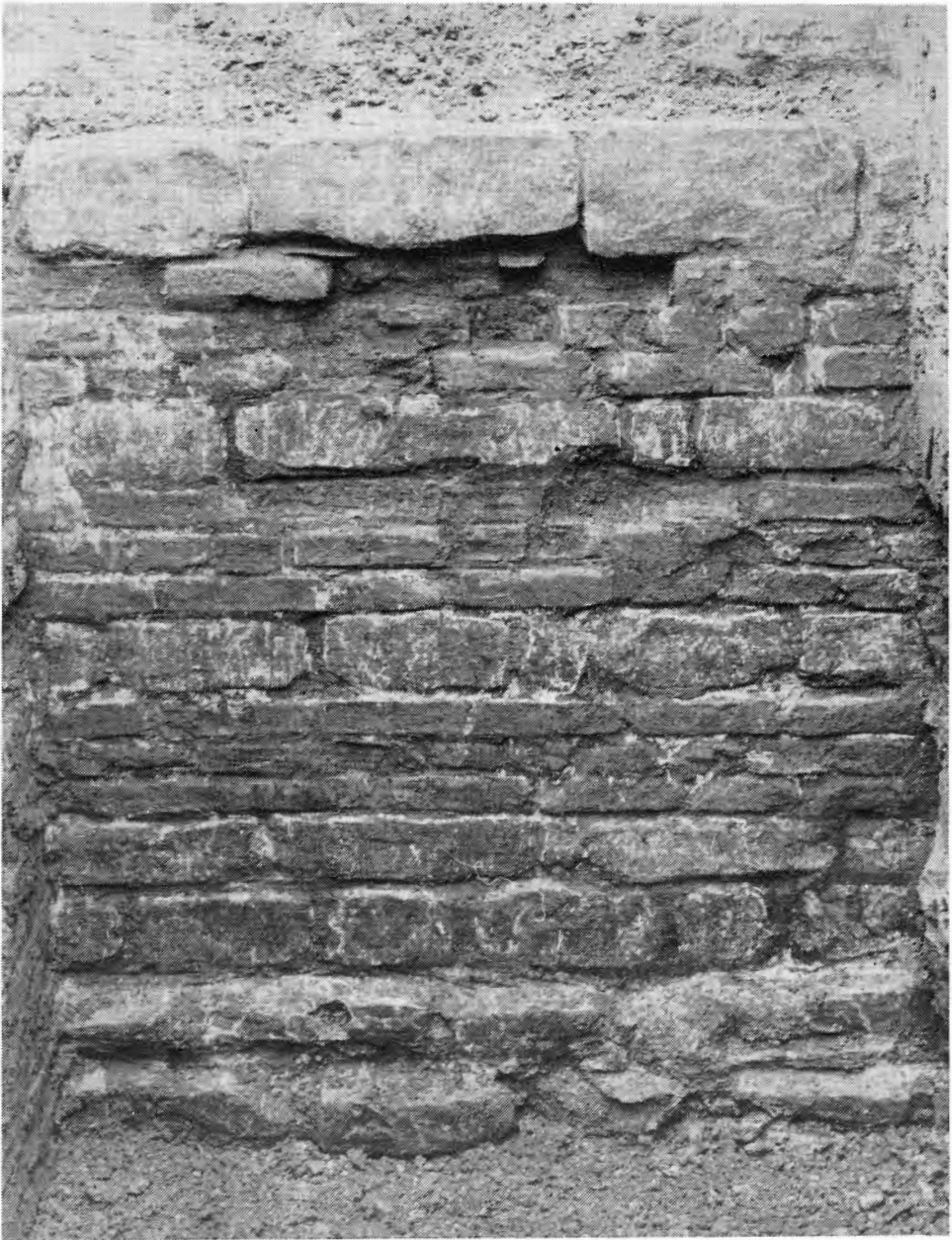
Detail van een vijftiende eeuwse gevel waarin men duidelijk de speklagen of lagen in witte zandsteen bemerkt. Deze muur stond in 't water van de slotgracht. Hieruit kan men duidelijk afleiden dat deze waterburcht in Brabantse gotiek gebouwd werd (afwisselend lagen witte zandsteen en baksteen).
